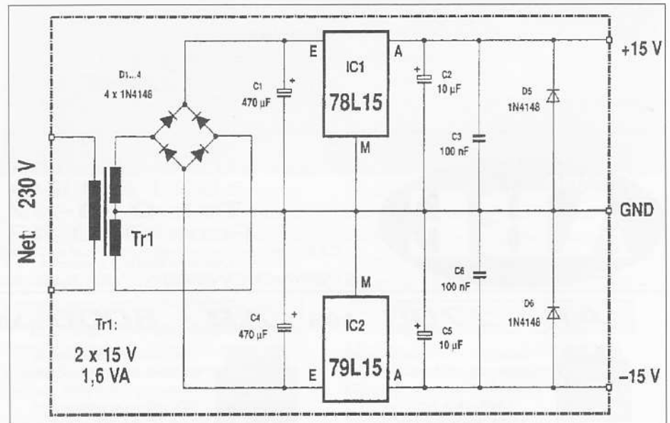
Schema voeding 2x50 mA.
